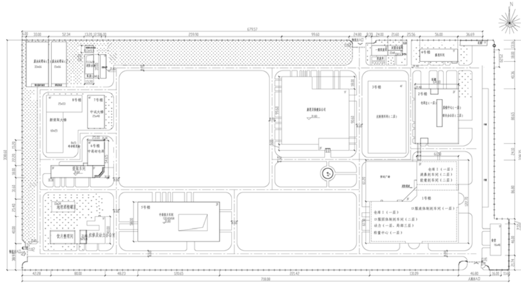
图 3.4 平面布局图
