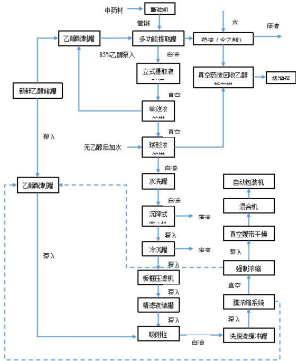
图 3.3 工艺流程图
